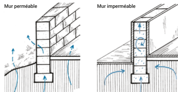
Mur perméable L'humidité transite librement et s'évacue
